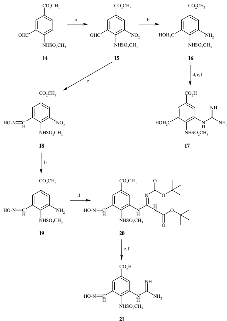
Scheme 2. Reagents and conditions: (a) fuming \text{HNO}_3 ; (b) \text{PtO}_2 , \text{H}_2 ; (c) \text{NH}_2\text{OH} , \text{HCl} ; (d) \text{BocHNC(=S)NHBoc} , \text{TEA} , \text{HgCl}_2 , \text{DMF} ; (e) \text{CF}_3\text{CO}_2\text{H} , \text{CH}_2\text{Cl}_2 ; (f) (1) \text{NaOH} , (2) \text{AcOH}/\text{H}^+ .
