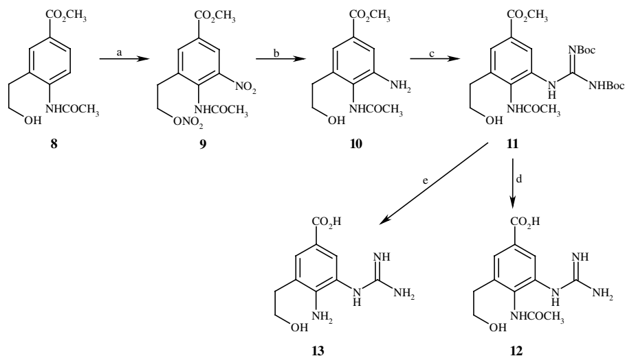
Scheme 1. Reagents and conditions: (a) fuming \text{HNO}_3 ; (b) \text{H}_2/\text{PtO}_2 , \text{MeOH} ; (c) \text{BocHNC(=S)NHBoc} , \text{TEA} , \text{HgCl}_2 , \text{DMF} ; (d) (1) \text{CF}_3\text{CO}_2\text{H} , \text{CH}_2\text{Cl}_2 ; (2) \text{NaOH} ; (3) \text{AcOH} ; (e) \text{HCl} .
