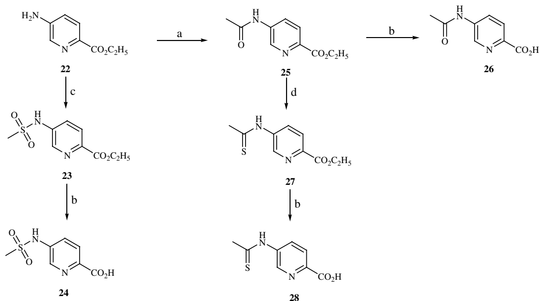
Scheme 3. Reagents and conditions: (a) \text{Ac}_2\text{O} , \text{AcOH} ; (b) \text{NaOH} , \text{H}^+ ; (c) \text{CH}_3\text{SO}_2\text{Cl} , pyridine; (d) Lawesson's reagent.
