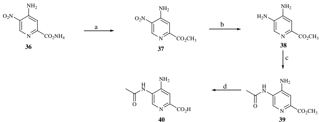
Scheme 5. Reagents and conditions: (a) MeOH, H 2 SO 4 ; (b) H 2 /PtO 2 ; (c) Ac 2 O, TEA; (d) NaOH, H + .
